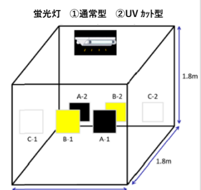
図1.試験室内の供試サンプルの配置
