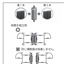
引分け用取手付開閉金具 (マグネット面詳細図)
